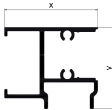
RGL72-B kg/m: 1.083
