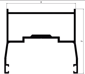
RGL72-F kg/m: 1.155
