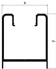
RGL72-D kg/m: 1.186
