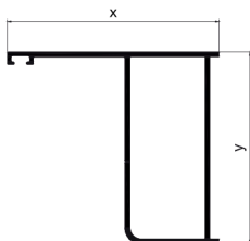
RGL72-G kg/m: 0.927
