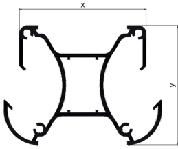
RGL70-A kg/m: 2.206
